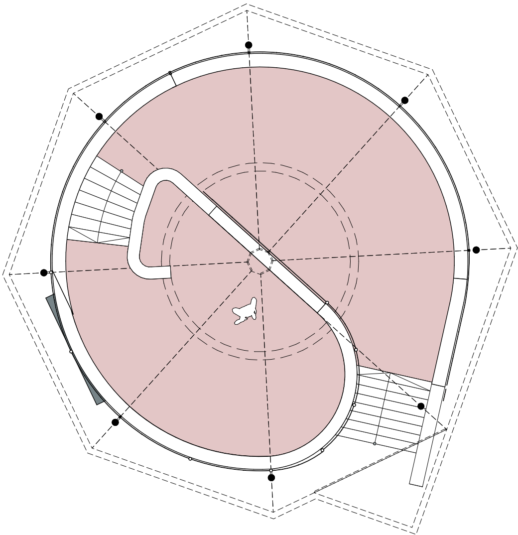
1e verdieping - 1:100
