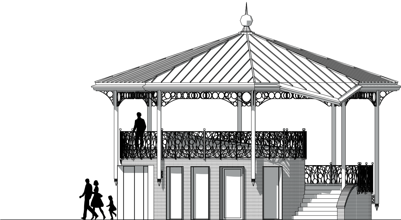
Voorgevel - 1:100
