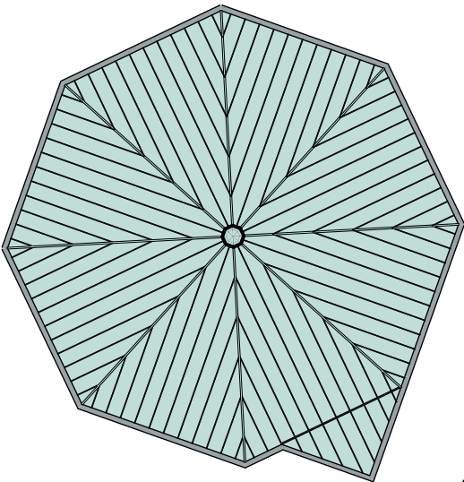
Dakaanzicht - 1:200
