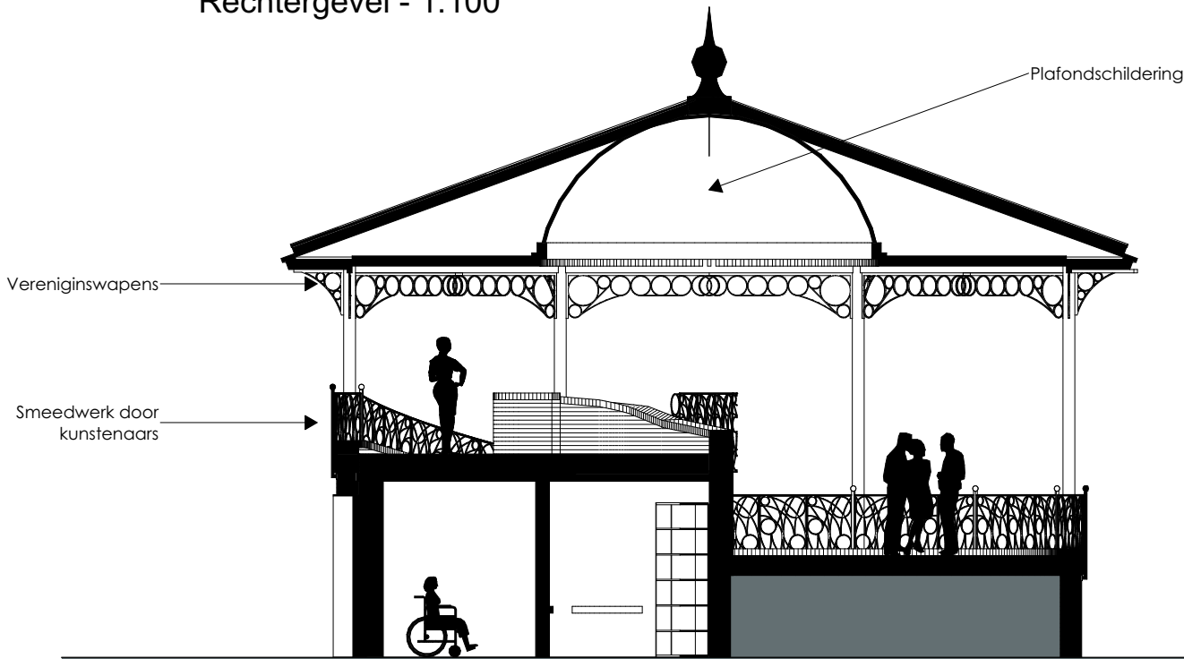
Rechtergevel - 1:100
